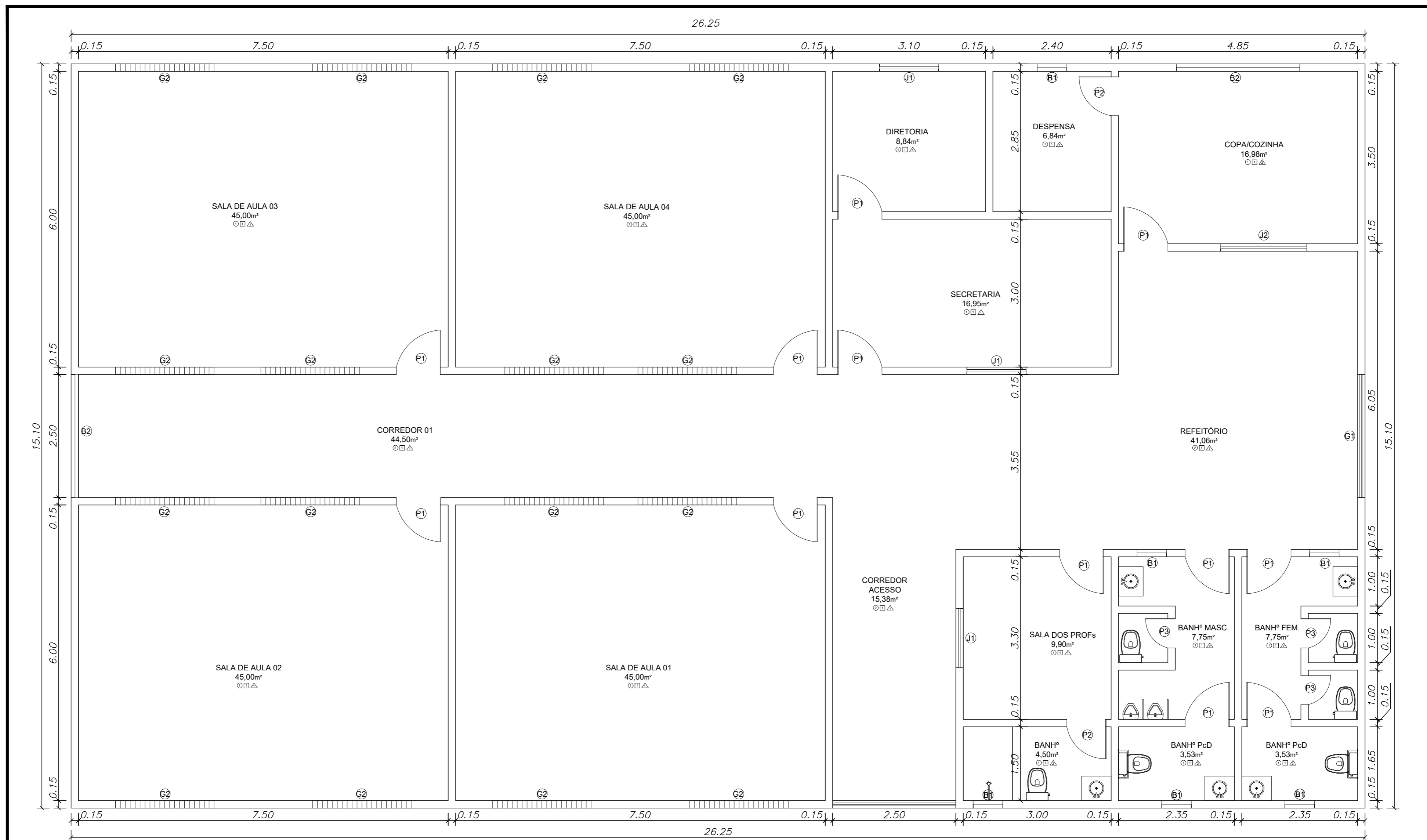
PLANTA BAIXA PROPOSTA DA ESCOLA BOA ESPERANÇA III - COMUNIDADE SÃO LOPES
